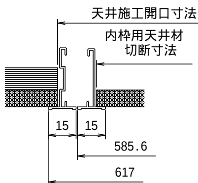
天井下地収まり図 ( 1 / 2 )
